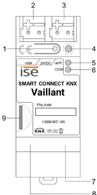
Abbildung 1: Geräteaufbau
